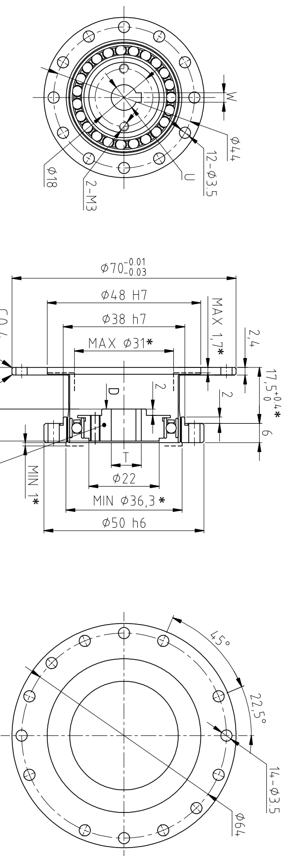
Wave generator-A
