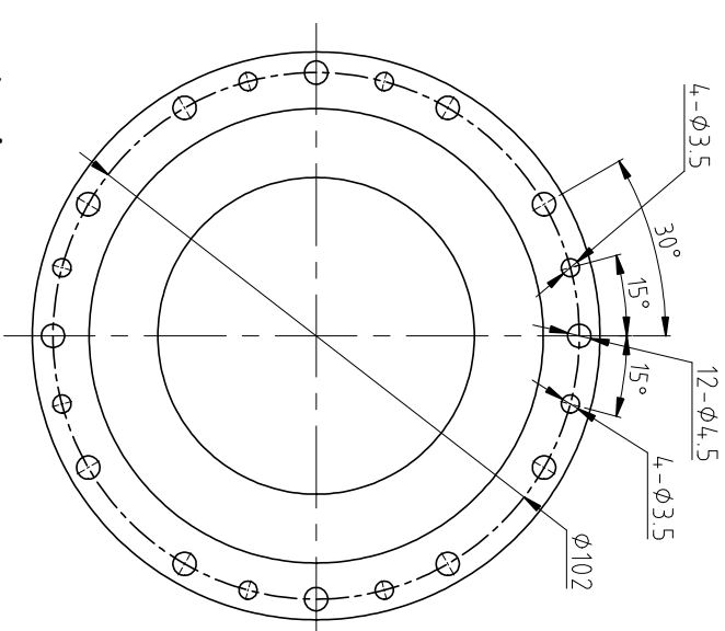
Wave generator-A
